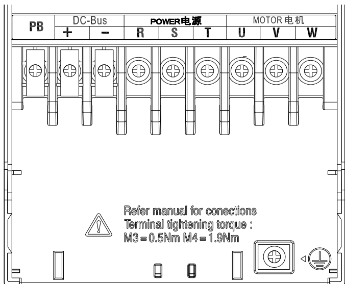
b) GS750-5R5-3B~GS750-022-3B
