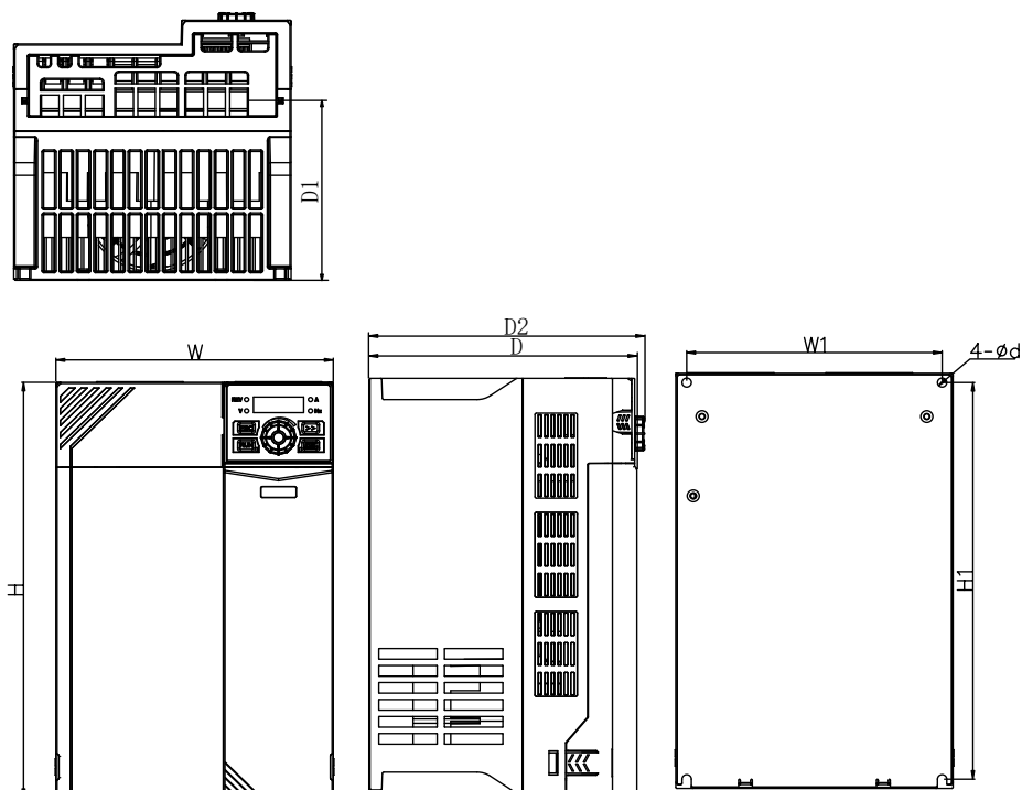
(a) Размеры моделей от GS750-0R7-3В до GS750-022-3В
