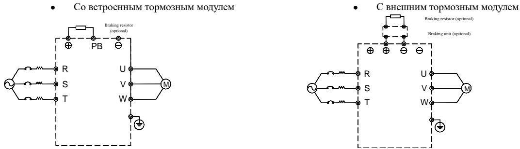
Рис.3-3 Стандартная схема подключения
