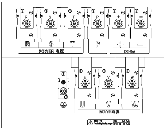
f) GS750-132-3~GS750-160-3
