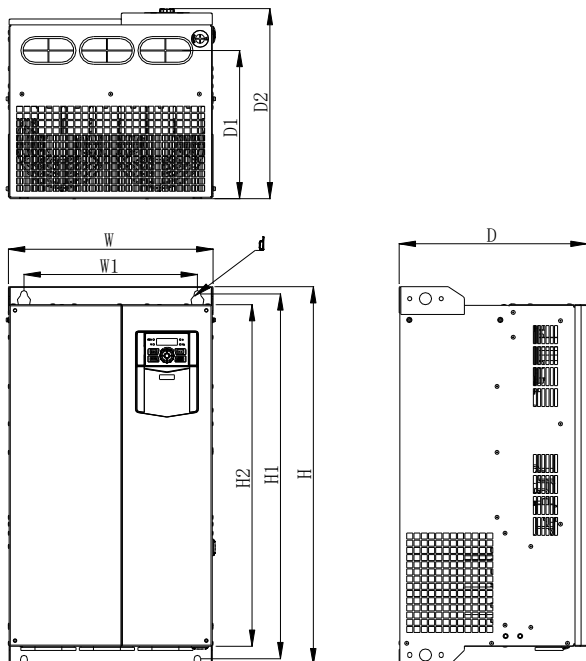
(с) Размеры моделей от GS750-090-3 до GS750-160-3
