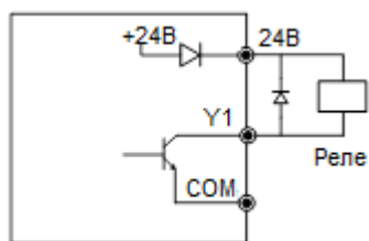
a: Со встроенным питанием NPN
