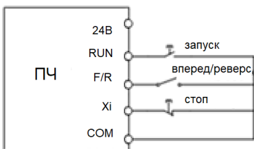
(b) Трехпроводное управление (F00.03=3)
