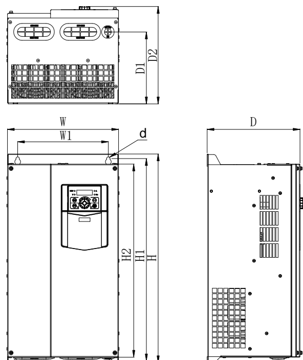
(b) Размеры моделей от GS750-030-3 до GS750-075-3
