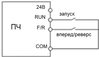
(a) Двухпроводное управление (F00.03=0)
