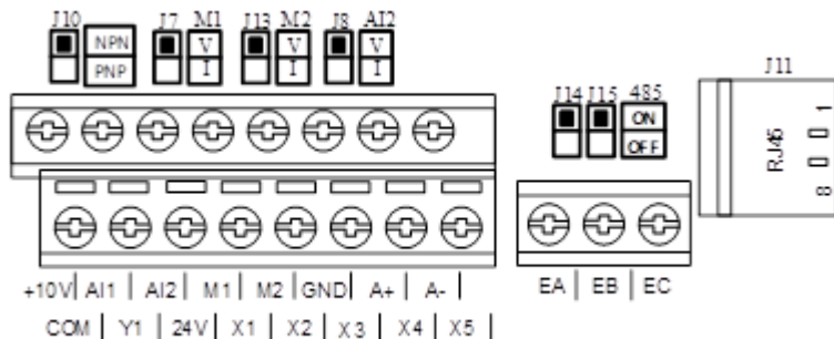
Рис.3-11 Расположение управляющих клемм 1
