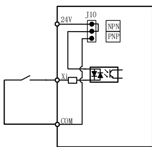
a: Со встроенным питанием в NPN режиме
