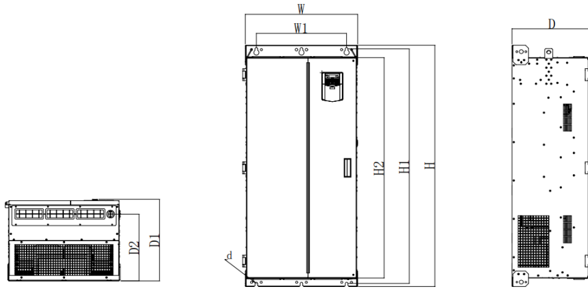
(f) Размеры моделей от GS750-280-3 до GS750-315-3
