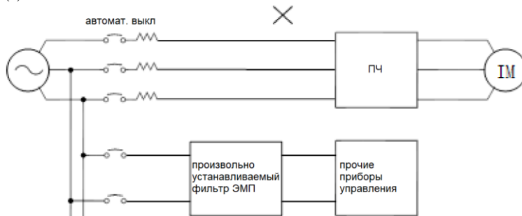
Рис. 3.6: Неправильная установка фильтра помех
