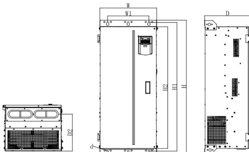
(d) Размеры моделей от GS750-185-3 до GS750-220-3
