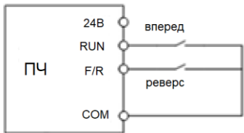
(c) F00.03=1 Двухпроводное управление
