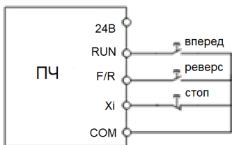
(a) Трехпроводное управление (F00.03=2)
