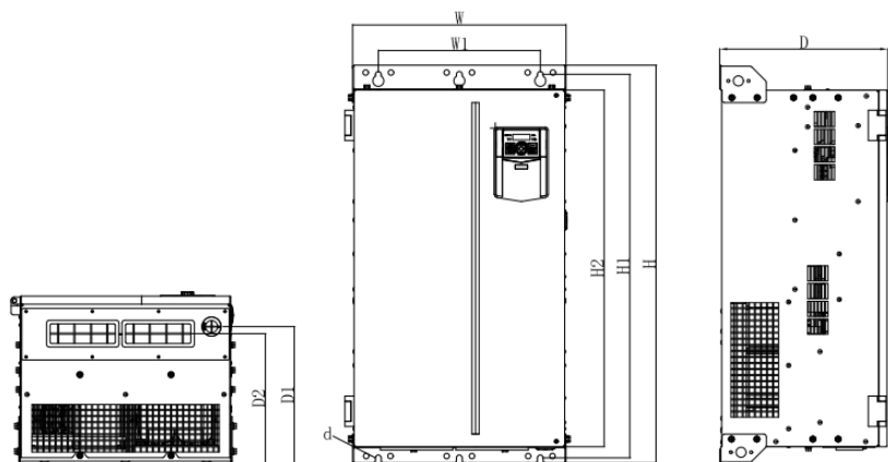
(d) Размеры моделей от GS750-185-3 до GS750-220-3
