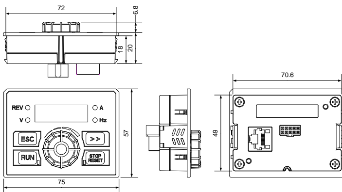
(h) Размер панели управления GS750
