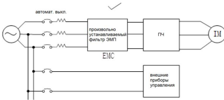
Рис.3-5 Корректная установка фильтра помех
