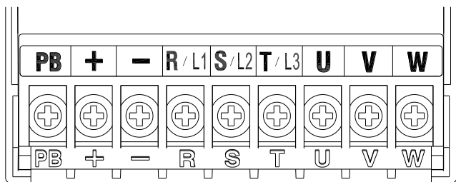
a) GS750-0R7-3B~GS750-1R5-3B
