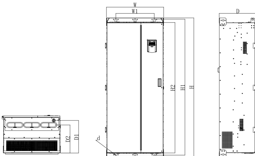
(g) Размеры моделей от GS750-355-3 до GS750-450-3
