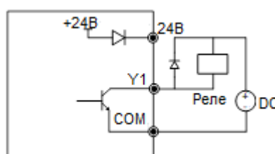
b: С внешним питанием NPN
