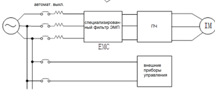
Рис.3-5 Корректная установка фильтра помех
