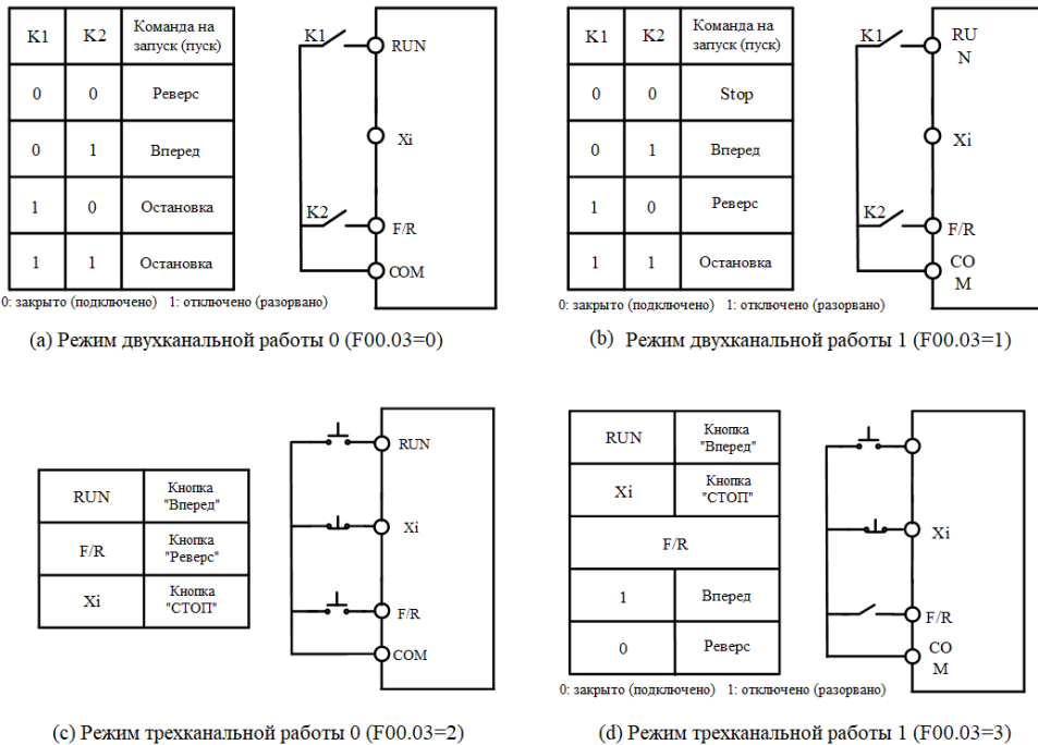
Рис. 1-6 Диаграмма логики управления входных клемм
